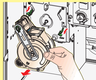
Fjern alle slanger, coveret foran bryggeren og kaffetrugten. Fjern bryggeren.
